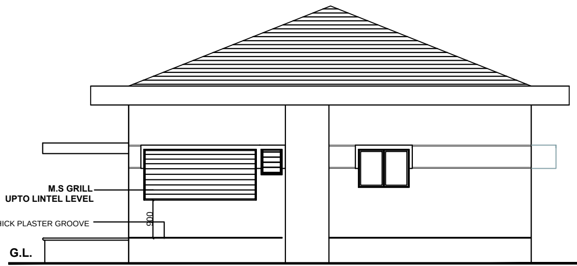
ELEVATION DD
